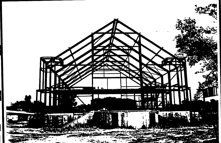
A frontal view showing the Church steel frames after erection. منظر امامي يـ الهياكل الحديدية الرئيسية لمبنى الكنيسة بعد تركيبها
